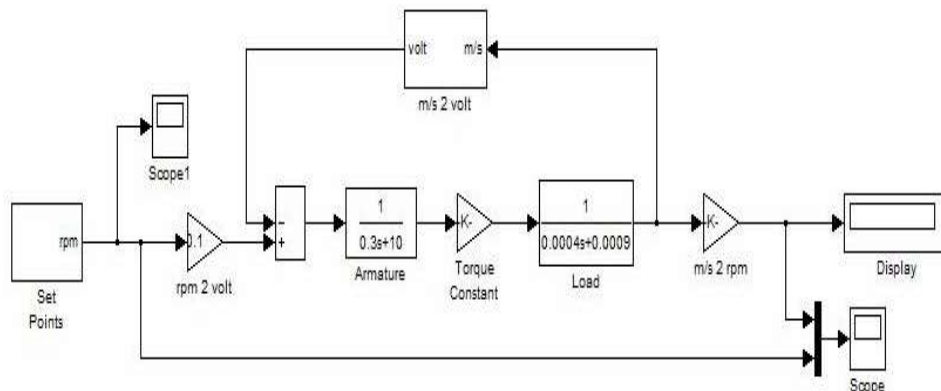
شکل ۱- شبیه سازی موتور الکتی AC با استفاده از نرم افزار MATLAB
