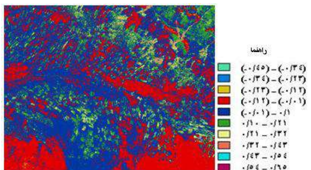
شکل 7: شاخص گیاهی IR2
