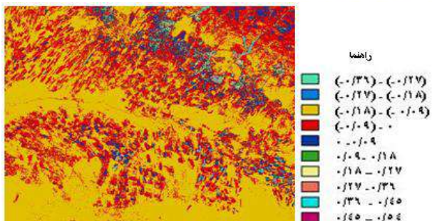
شکل 3: شاخص پوشش گیاهی NDVI
