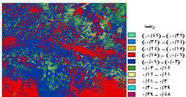
شکل 5: شاخص گیاهی IR1
