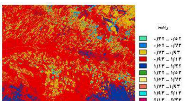
شکل 8: شاخص گیاهی Moisture Stress Index
