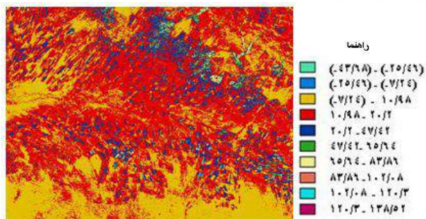
شکل 4: شاخص پوشش گیاهی GVI
