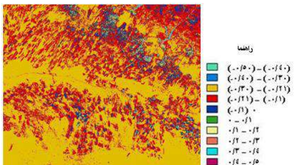
شکل 9: شاخص گیاهی Modified Normalized Index
