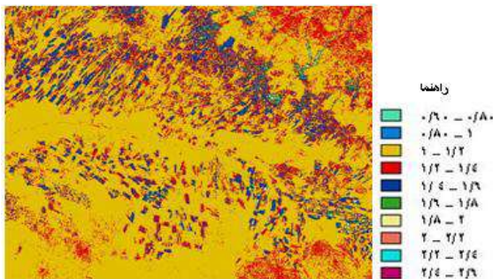
شکل 6: شاخص پوشش گیاهی Leaf Water Index
