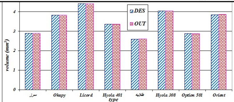
شکل ۸: نزدیکی ارقام حاصل از پیش‌بینی به وسیله شبکه‌های عصبی با مقدار واقعی برای ۸ گونه دانه کلزا
