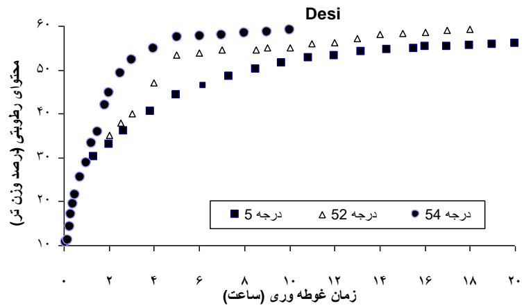
شکل ۱. مشخصات جذب رطوبت توسط انواع نخودهای مورد آزمایش طی غوطه وری
