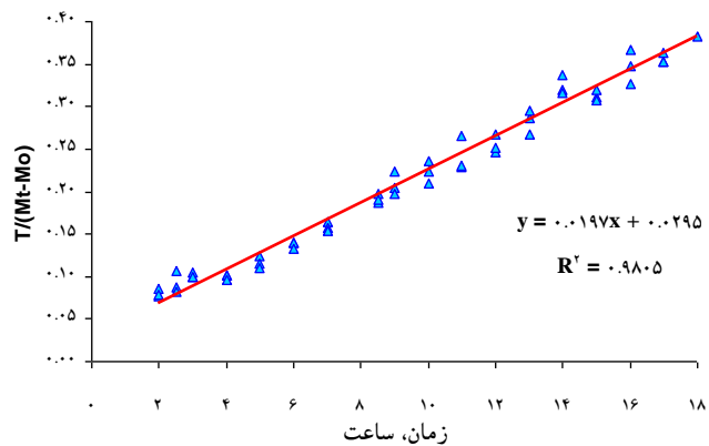
شکل ۲. منحنی خطی مدل Peleg در جذب رطوبت توسط نخود Desi طی شرایط غوطه وری
